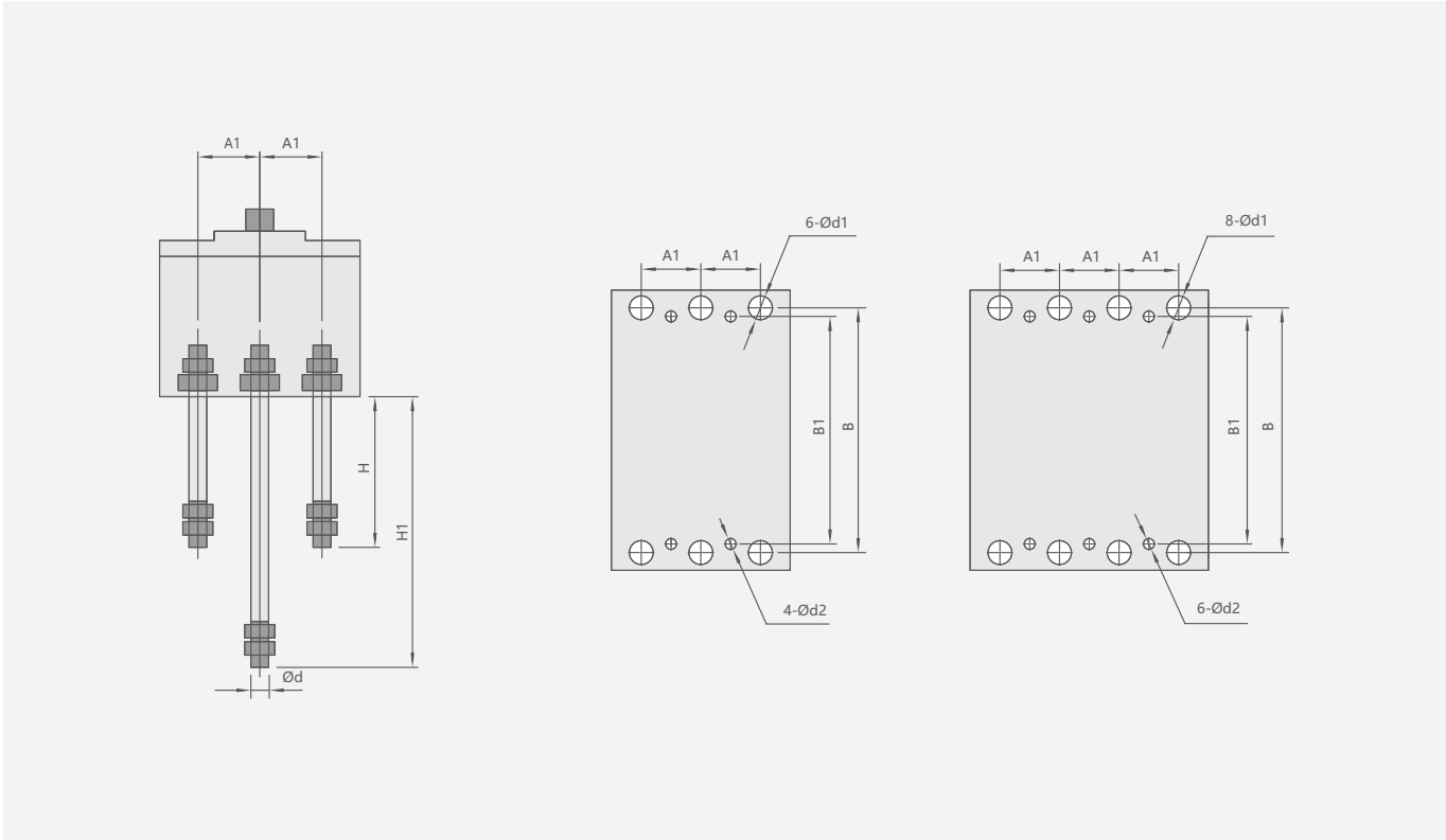
Габаритные и монтажные размеры (мм)
