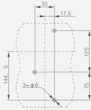
3P: монтаж на панель
