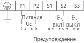
Схема подключения
