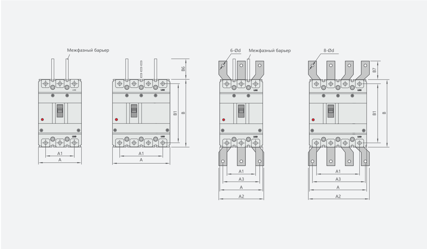
Габаритные и монтажные размеры (мм)
