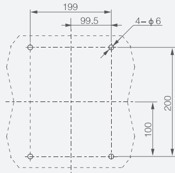
3P: монтаж на панель
