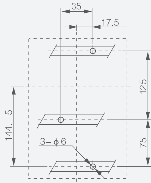
3P: монтаж на направляющие
