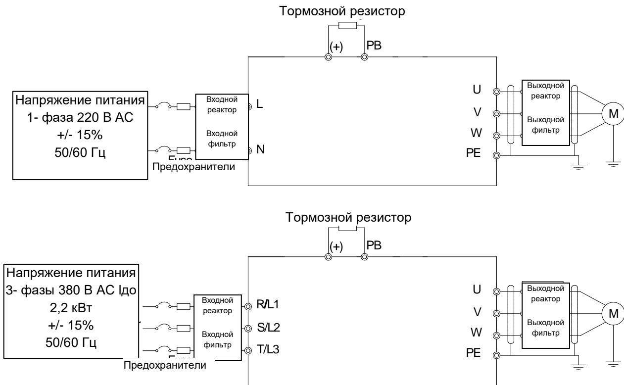
Рис. 5-3.1. Подключение силовых кабелей и управления
