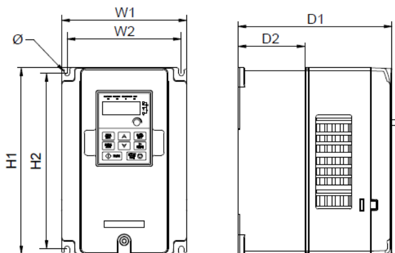
Рис. 4.8 Настенный монтаж 4 – 37 кВм
