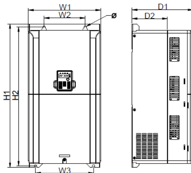
Рис. 4.8 Настенный монтаж 4 – 37 кВм
