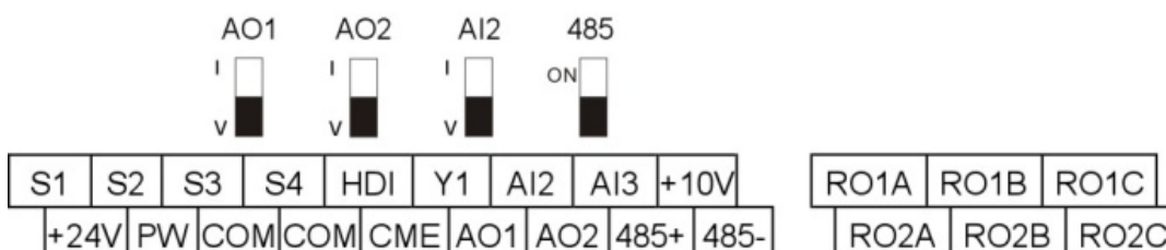
Рис. 5-17 Клеммы цепей управления
