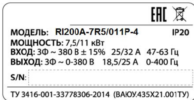
Рисунок 2-1. Шильдик преобразователей частоты GD200A
